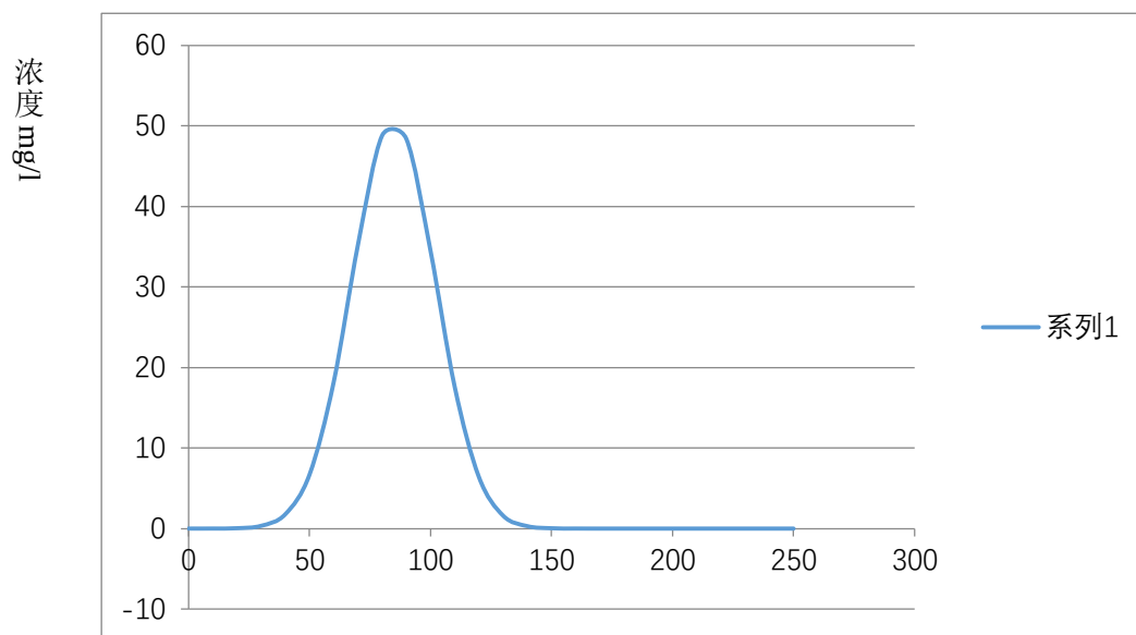
渗漏 1000 天后不同距离硫酸盐浓度变化预测图
