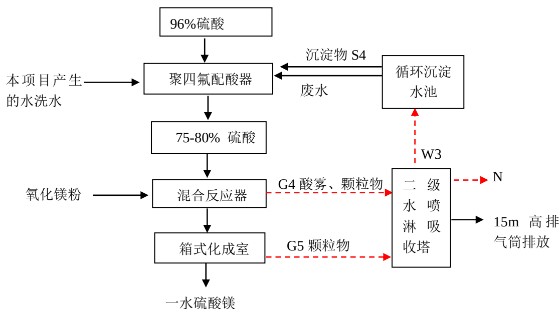
图 2.2-4 酸液综合利用生产工艺流程图
