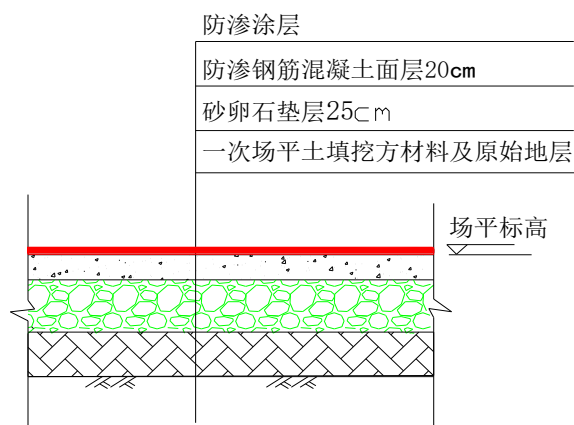
图 5.1-3 重点污染防治区典型防渗结构示意图
