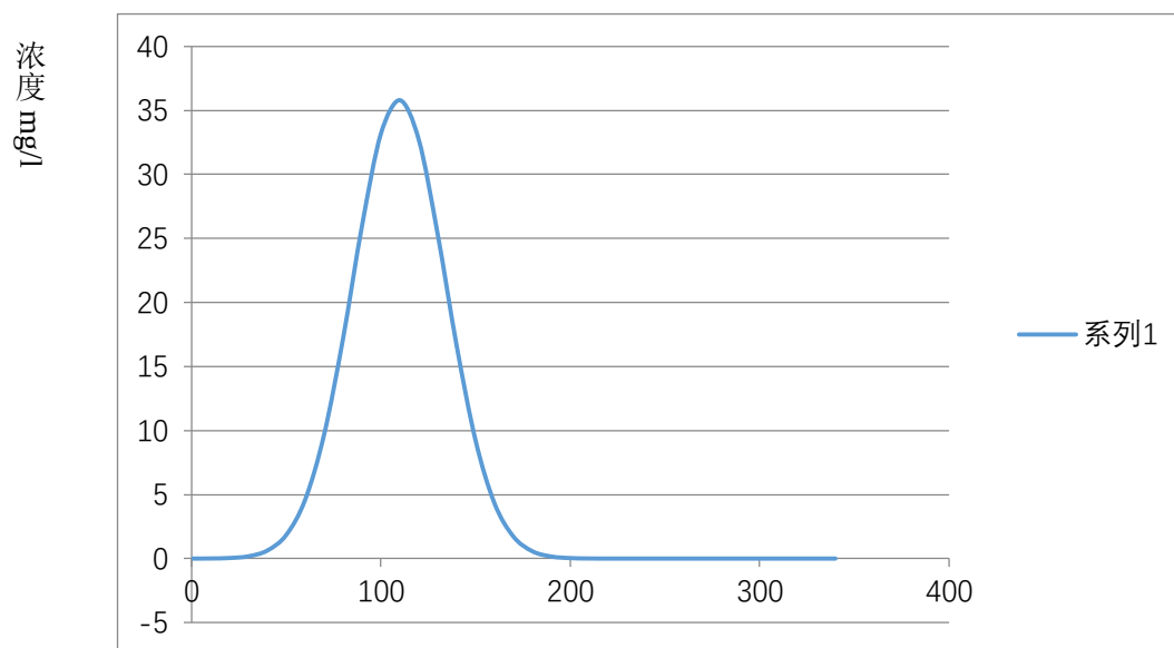
渗漏 2000 天后不同距离硫酸盐浓度变化预测图
