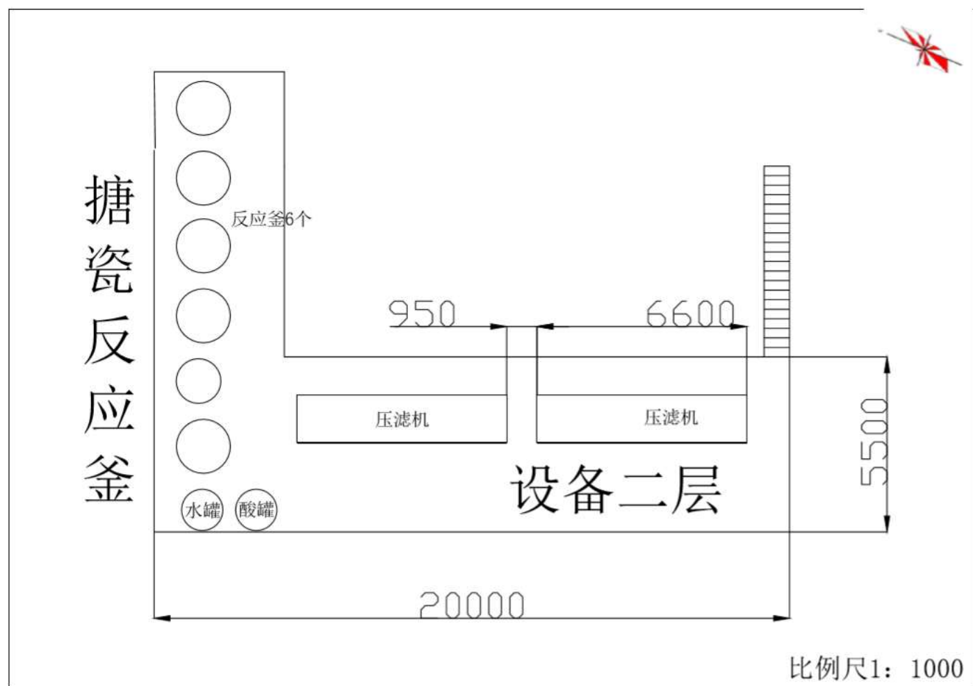
图2.2-2 车间二层设备平面布置图
