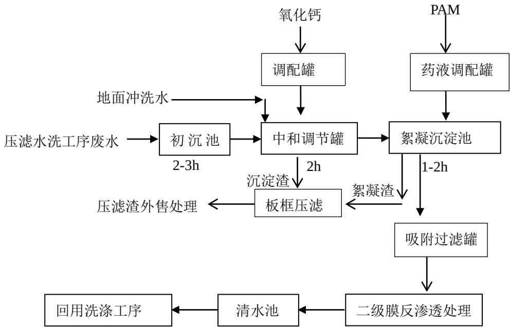
图 5.1-1 废水处理工艺流程图
