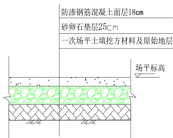
图 5.1-2 一般污染防治区典型防渗结构示意图
