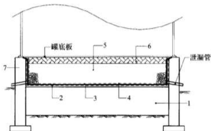
图 5.1-4 罐基础高密度聚乙烯(HDPE)膜防渗层示意图
