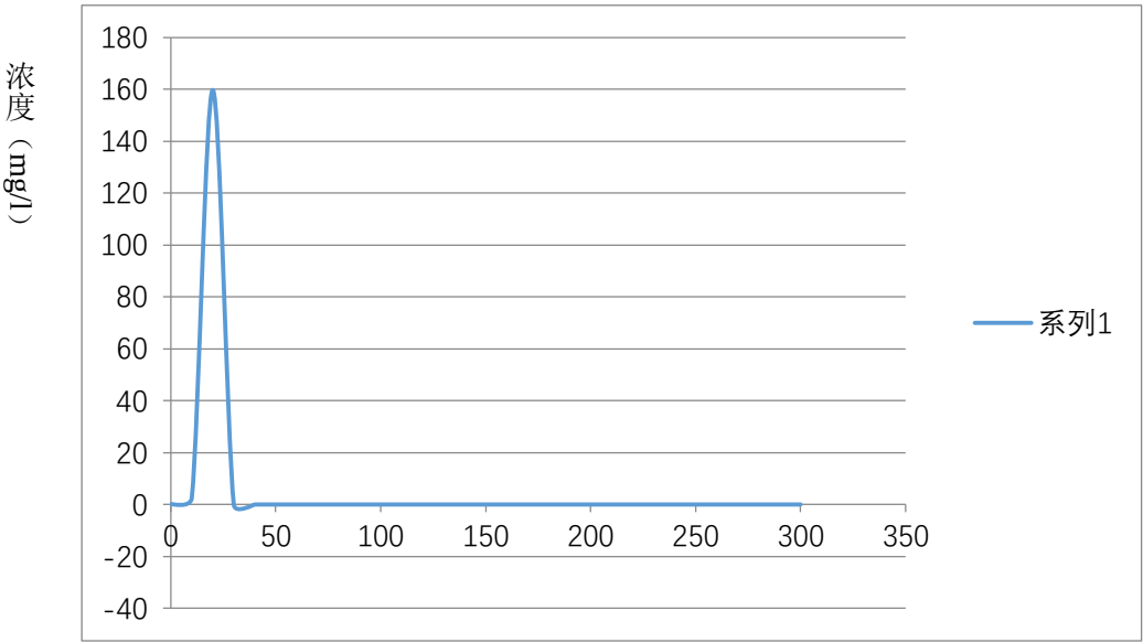
渗漏 100 天后不同距离硫酸盐浓度变化预测图
